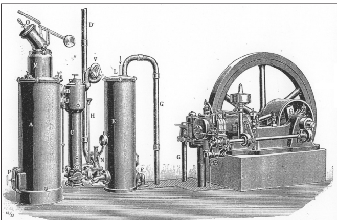
Gaskraftanlage wie in der Kaschützühle Hohenmölsen
