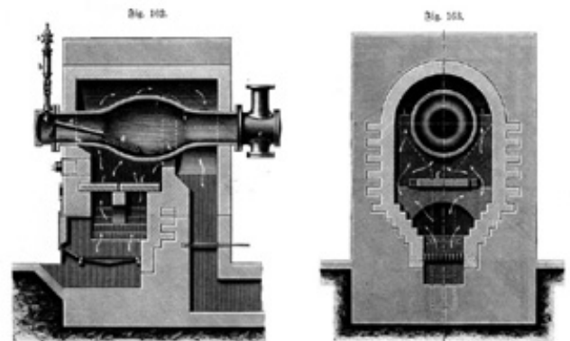
Schnittzeichnung eines Retortenofens
