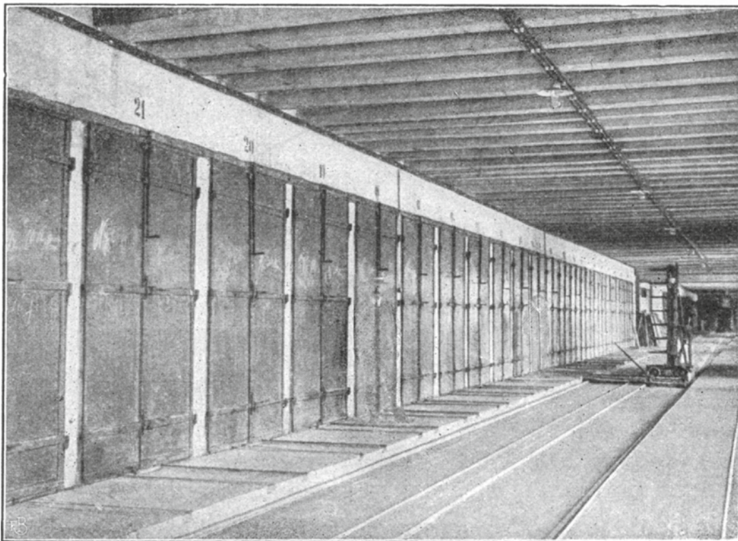
Schiebebühnenraum vor einer Kammertrocknerei; Quelle: Handbuch der Ziegeleitechnik, Weber, 1914
