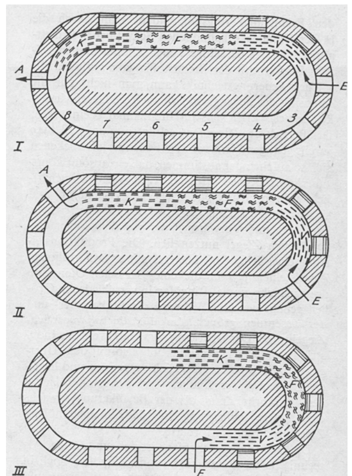
Abb. 7.4. Die Betriebsweise eines Ziegelringofens in einer schematischen Darstellung dreier Ablaufstadien (I, II, III)
