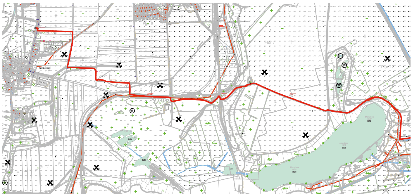
Trassenverlauf Neubau Fernwärmeleitung Zembschen - Profen
