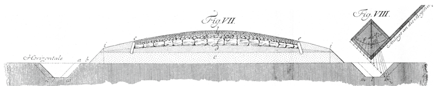
Skizze (Ausschnitt): Profilzeichnung einer befestigten Kiesstraße mit Winkelmaß für Böschungen von 1781
