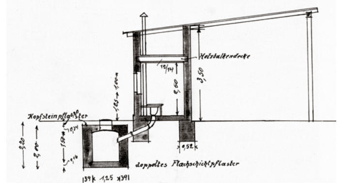
Bauzeichnung zum Einbau der Toilette 1912
