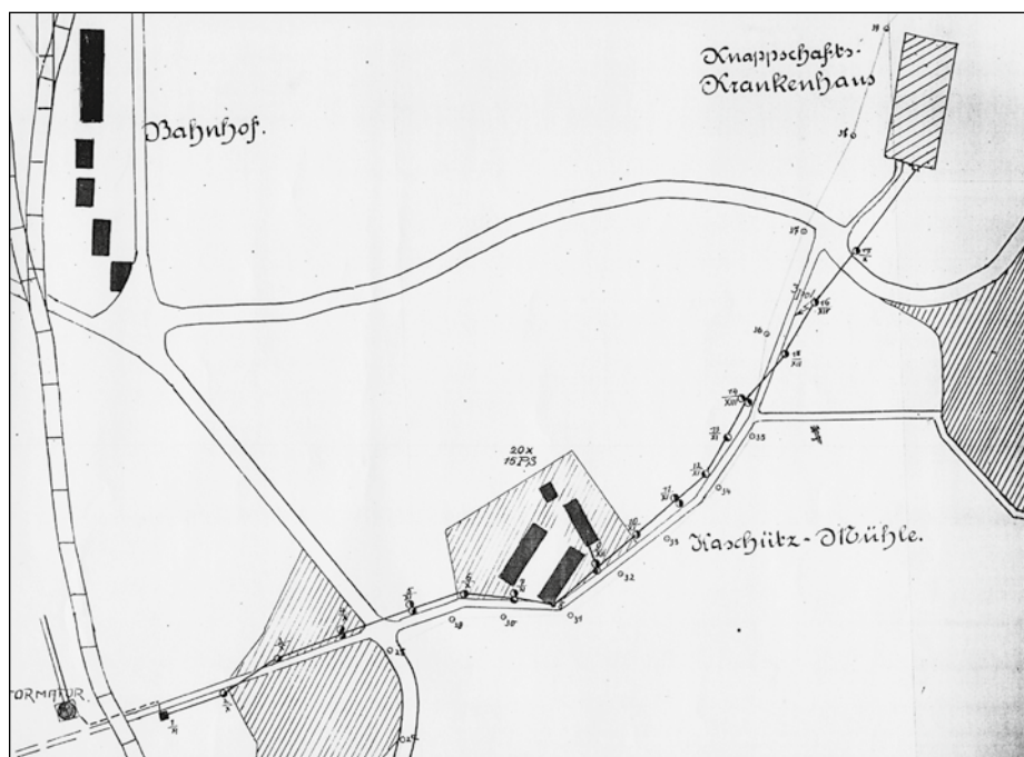
Lageskizze der Freileitung vom Trafوهاus nach der Kaschütz-Mühle und dem Krankenhaus
