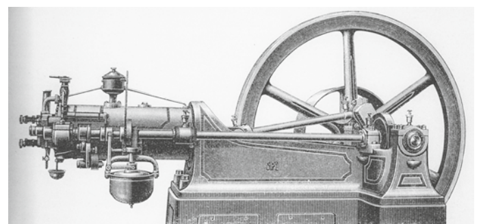
Liegender Otto-Motor mit Schiebersteuerung
