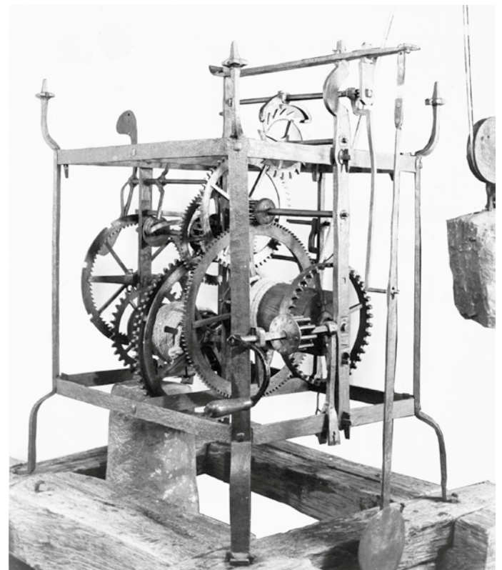
Turmuhrwerk von 1519, ähnlich dem auf dem Kirchturm Hohenmölsen (Aus Turmuhrwerke von Bernhard Schmidt, Deutsche Gesellschaft für Chronometrie e.V.)
